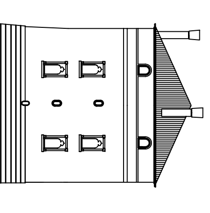
PROSPETTO OVEST
