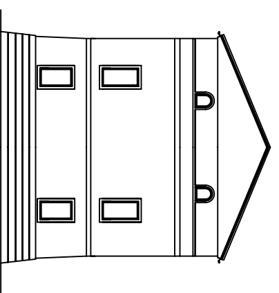
PROSPETTO EST
